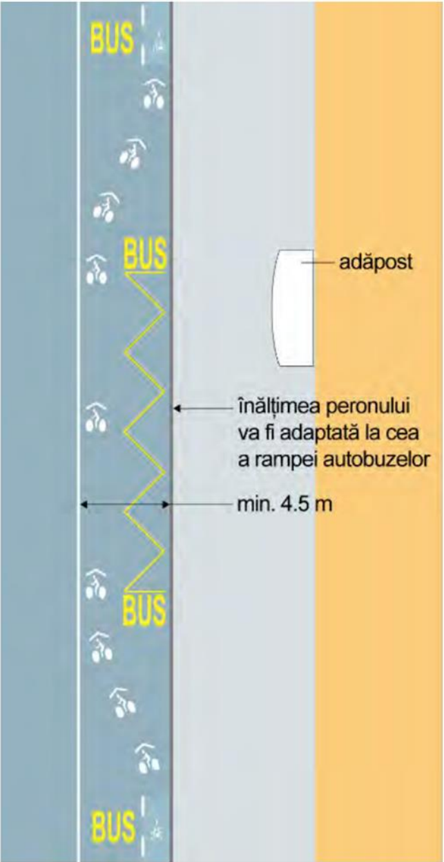
Figură 6-36 - Configurarea unui traseu de benzi ciclabile în proximitatea unei stații de transport public (preluare Ghid MDLAP/OPTAR)
