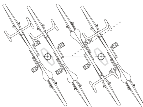
Figură 7-53 - Configurarea parcajului de biciclete pe rastel la 0° respectiv 45°
