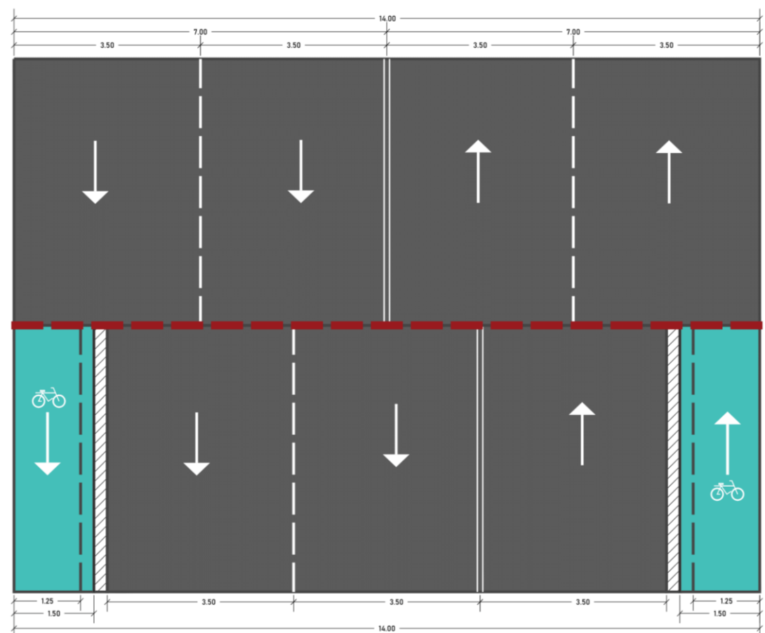
Figură 6-17 - Plan de configurare a unui profil stradal de 14m cu diminuarea numărului de benzilor auto și configurație de infrastructură velo unidirecțională
