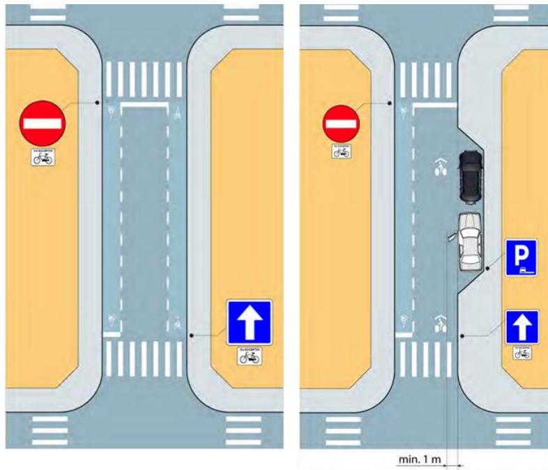
Figură 6-1 - Exemple de străzi cu sens unic în circulația bicicletelor permisă în dublu sens (preluare Ghid OPTAR)
