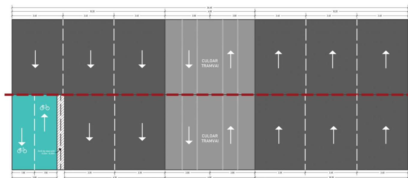
Figură 6-31 - Plan de configurare a unui profil stradal de 26,40 m cu reducerea numărului benzilor auto și configurarea unei infrastructuri velo bidirecțională principală
