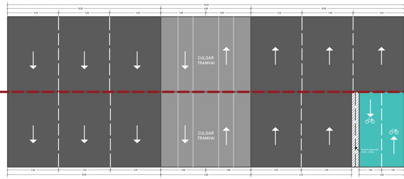
Figură 6-31 - Plan de configurare a unui profil stradal de 26,40 m cu reducerea numărului benzilor auto și configurarea unei infrastructuri velo bidirecțională principală
