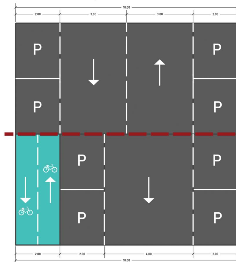
Figură 6-15 - Plan de configurare a unui profil stradal cuprins între 9m și 10m cu restructurarea circulației auto și configuare de infrastructură velo bidirecțională
