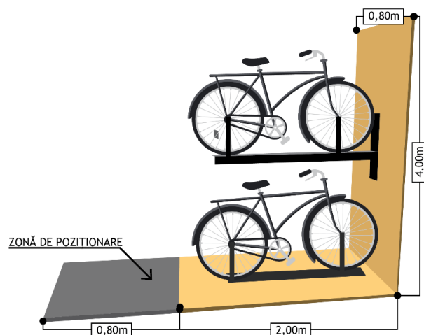
Figură 7-58 - Dotare parcaj modular cu sistem de parcare orizontală pe nivele a bicicletelor
