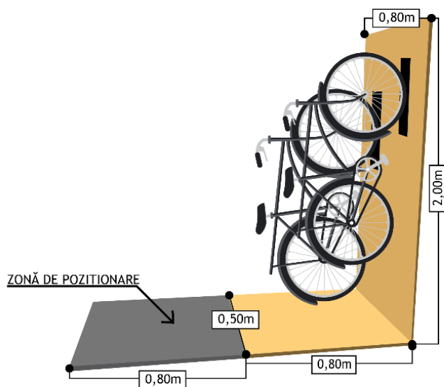
Figură 7-57 - Dotare parcaj modular cu sistem de parcare verticală a bicicletelor
