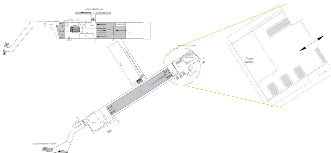
Figură 7-38 - Configurarea unui parcaj de biciclete în proximitatea accesului din cadrul stației de metro de la Piața Unirii 2
