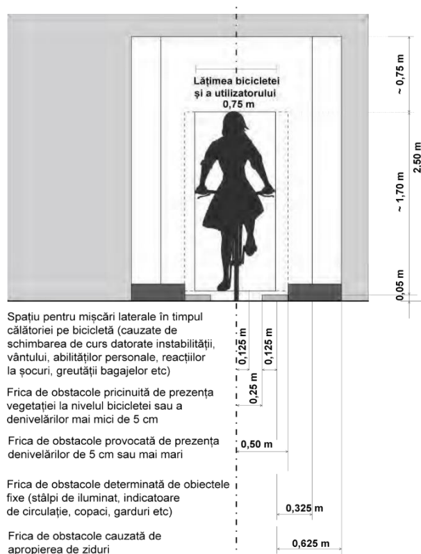
Figură 1-10 - Extras din ghiul OPTAR: distanțe față de obstacolele din vecinătate
