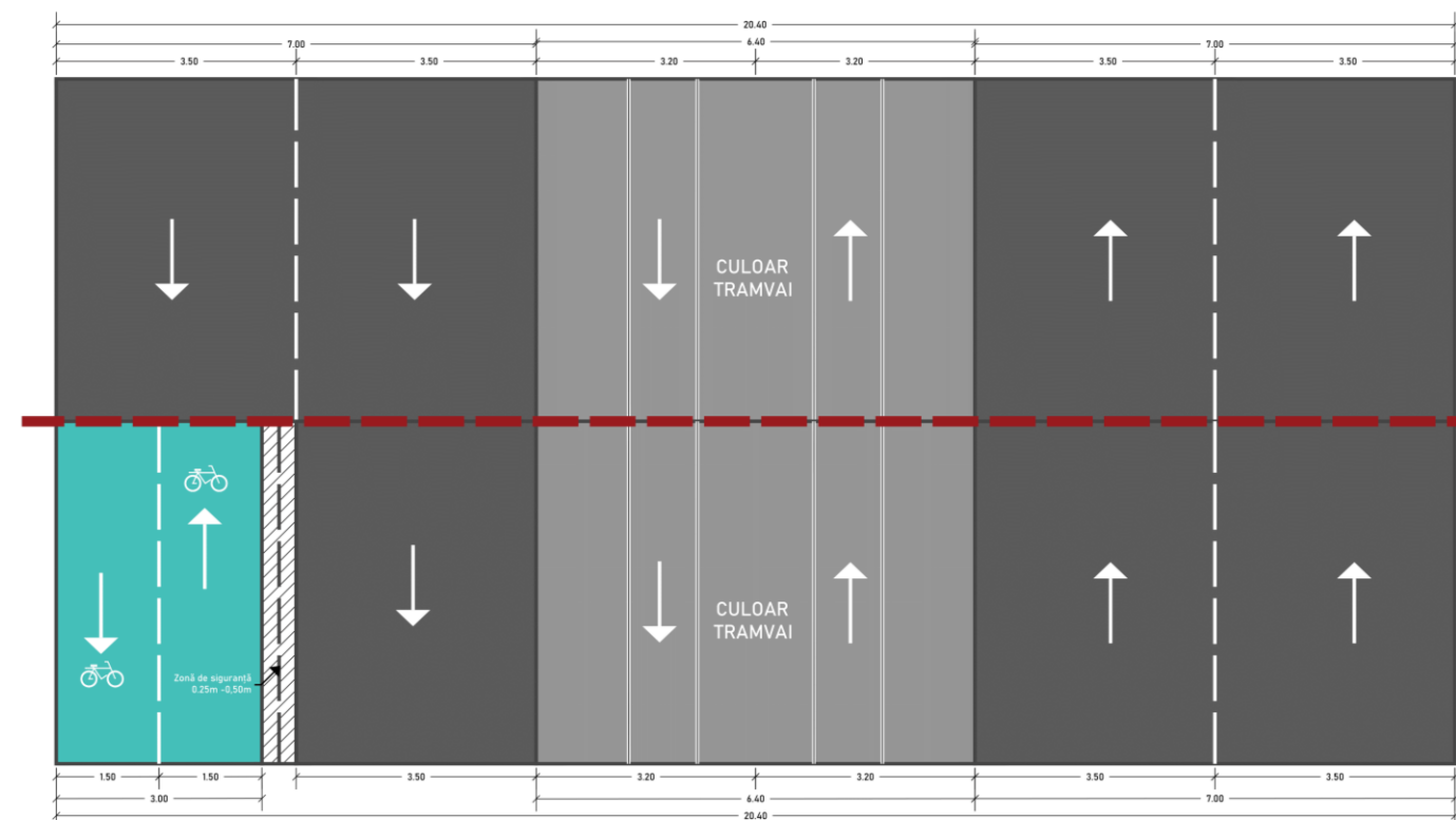
Figură 6-28 - Plan de configurare a unui profil stradal între 20,4 m cu diminuarea benzilor auto și configurarea unei infrastructuri de biciclete bidirecționale respectiv unidirecționale
