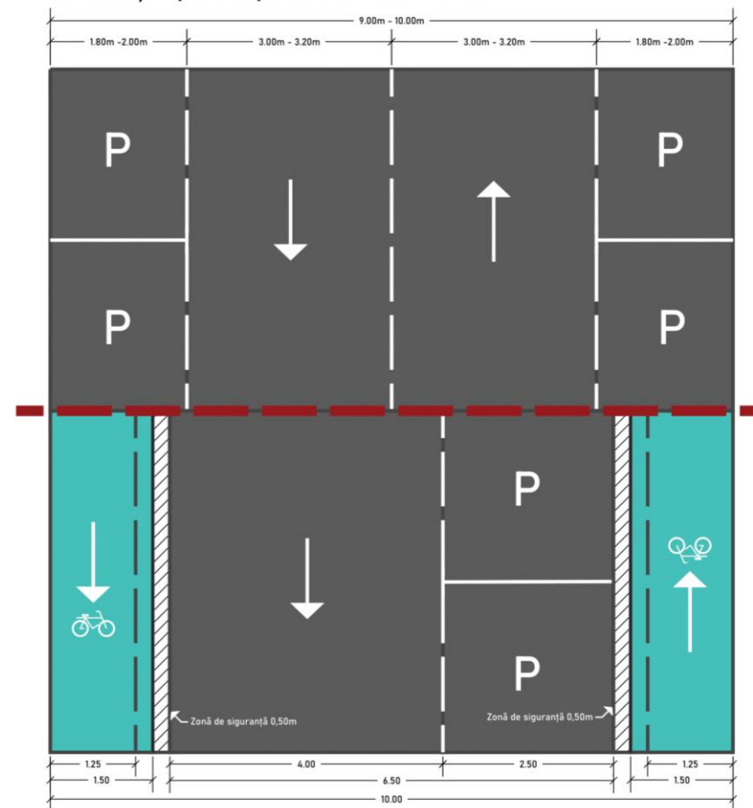
Figură 6-14 - Plan de configurare a unui profil stradal cuprins între 9m și 10m cu restructurarea circulației auto și confiugrare de infrastructură velo bidirecțională respectiv unidirecțională
