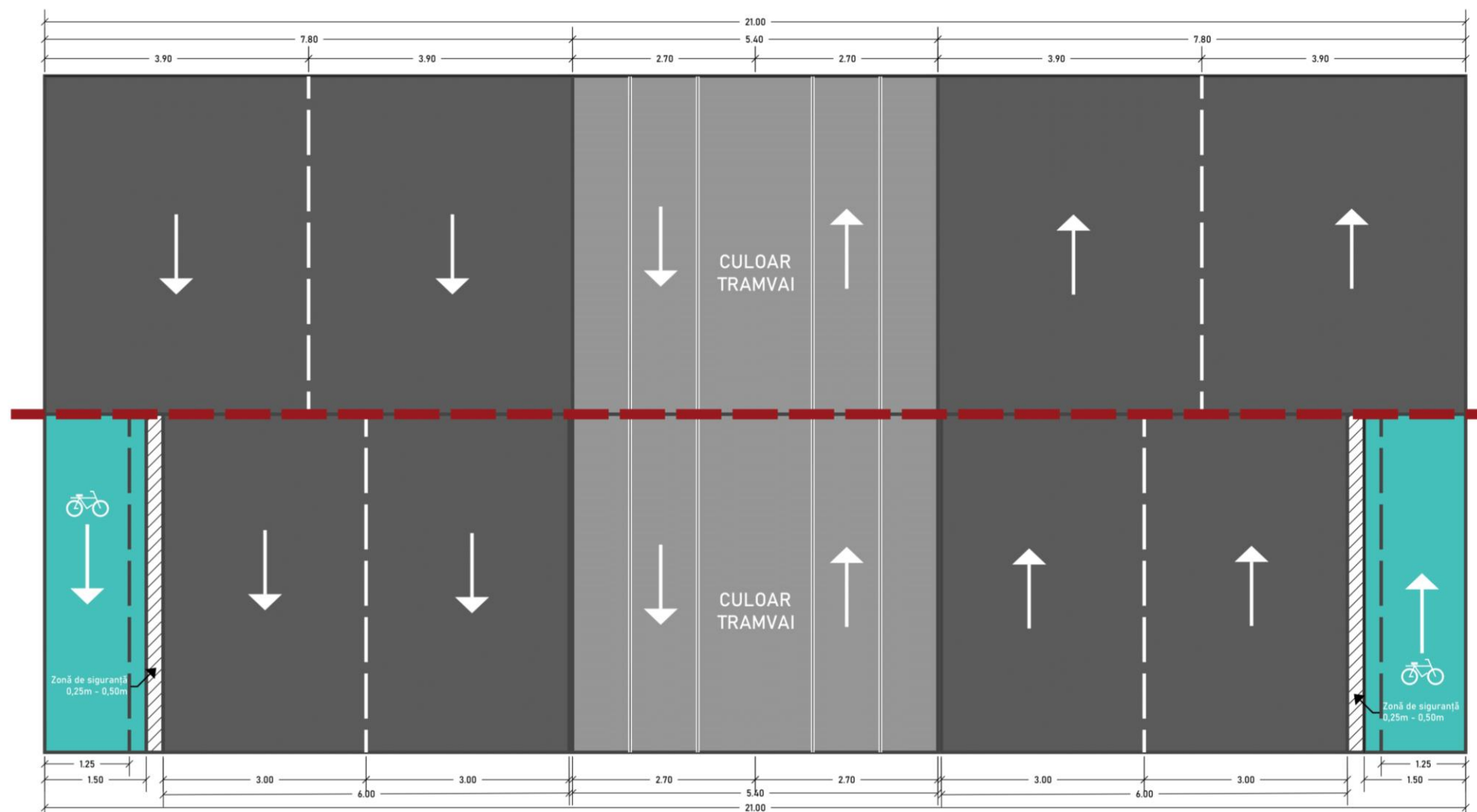
Figură 6-30 - Plan de configurare a unui profil stradal de 21m cu redimensionarea benzilor auto și configurarea unei infrastructuri velo unidirecționale principale
