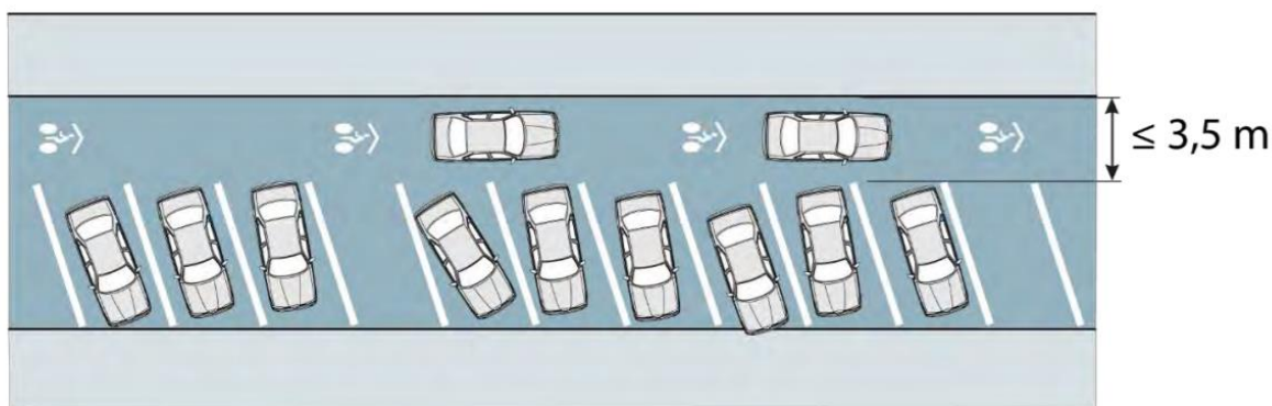
Figură 6-8 - Exemplu de marcaj pentru traseu sugerat pe străzi cu circulație auto în sens unic sau în interiorul alveolelor de parcare din afara zone de circulație auto (preluare Ghid OPTAR/MDRAP)
