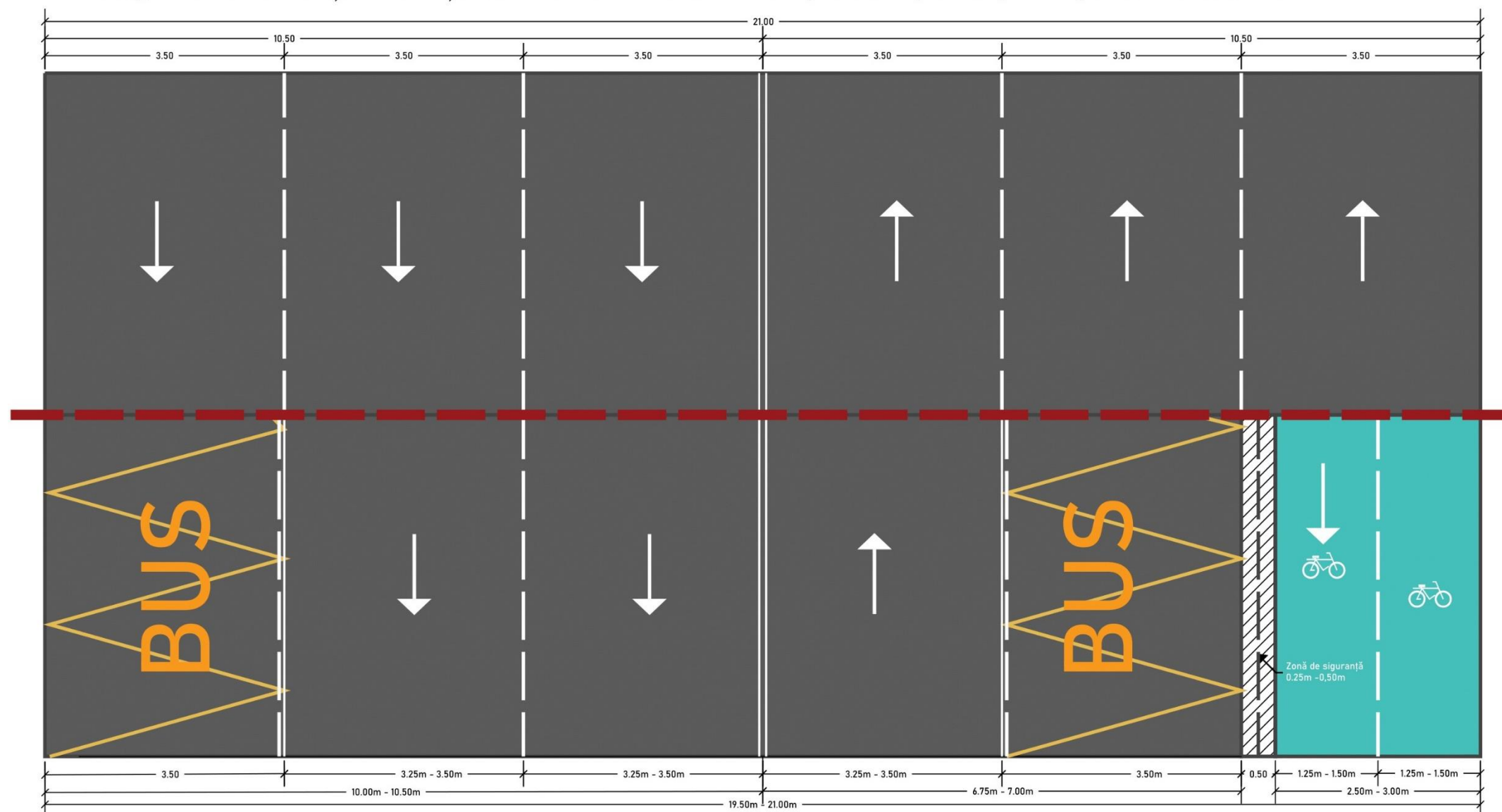
Figură 6-22 - Plan de configurare a unui profil stradal între 21m cu diminuarea, redimensionarea benzilor auto și configurație de infrastructură velo bidirecțională
