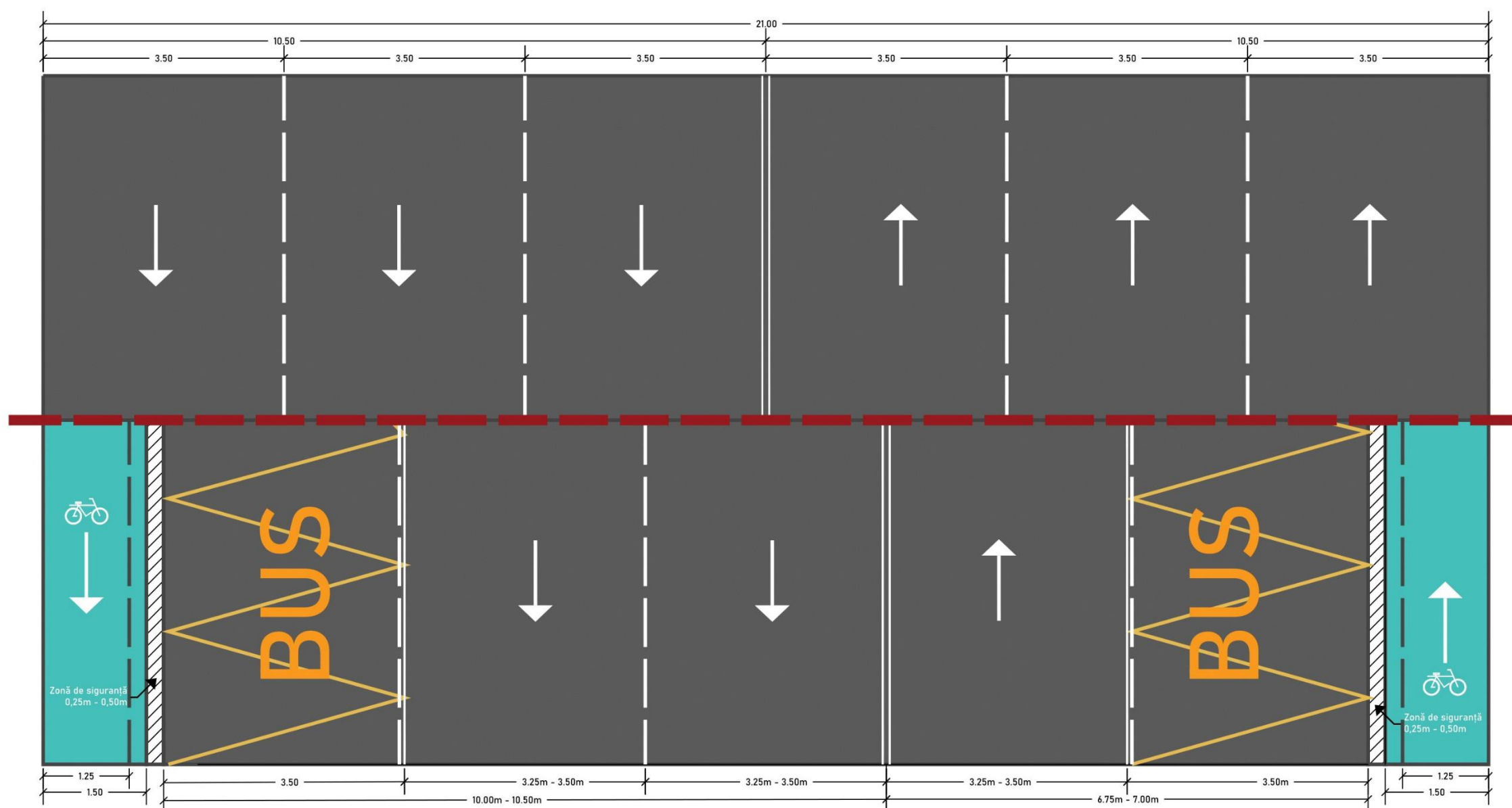
Figură 6-24 - Plan de configurare a unui profil stradal între 21m cu diminuarea, redimensionarea benzilor auto și confiugrare de infrastructură velo unidirecțională
