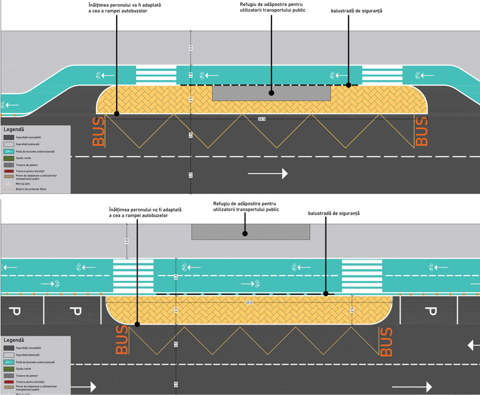
Figură 6-35 - Configurarea unui traseu de piste de biciclete în proximitatea unei stații de transport public
