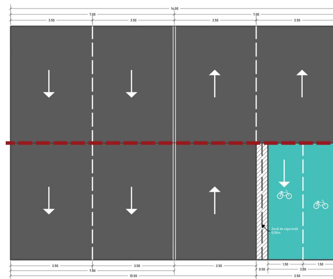
Figură 6-16 - Plan de configurare a unui profil stradal de 14m cu diminuarea numărului de benzi auto și configurație de infrastructură velo bidirecțională
