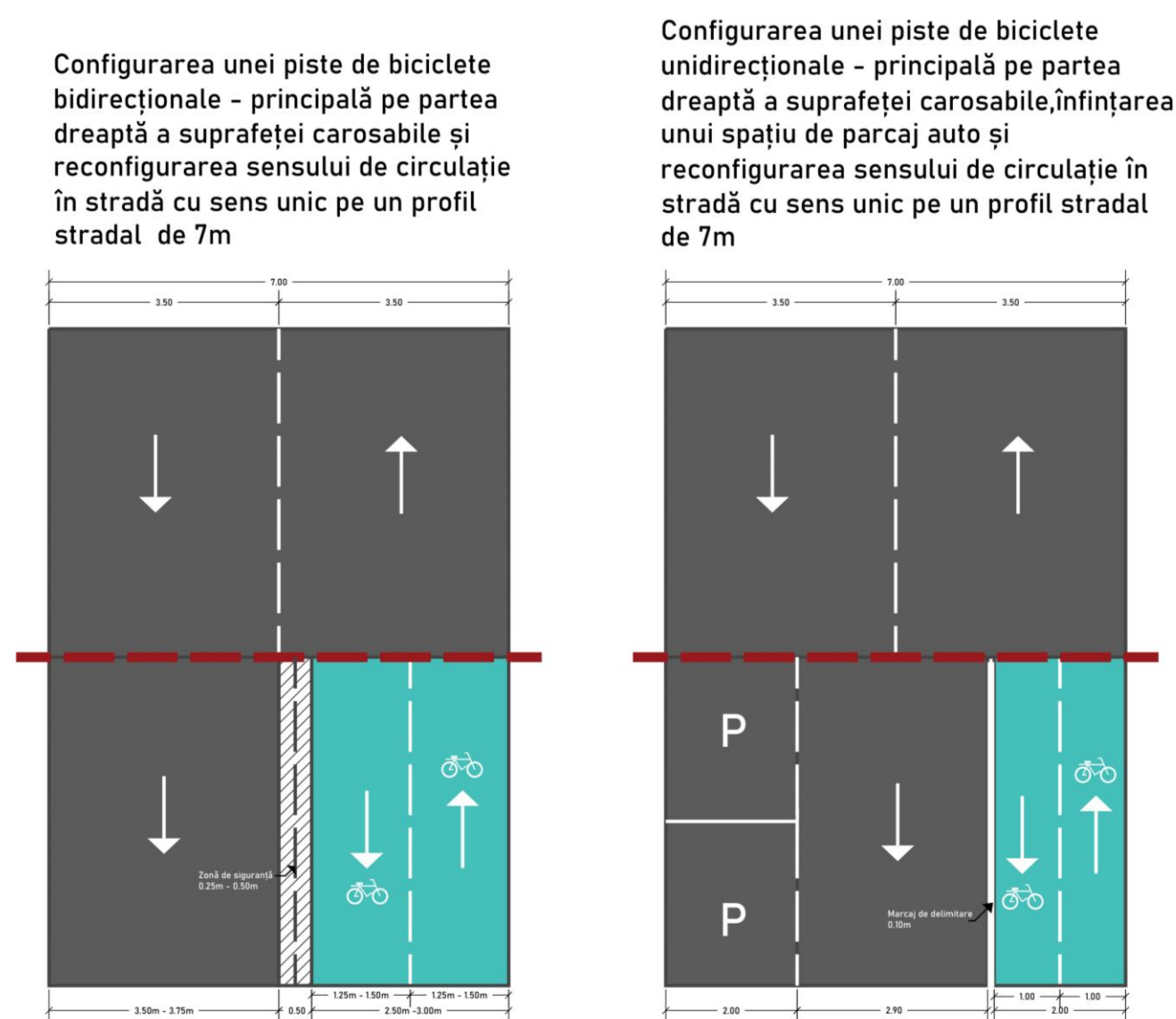
Figură 6-12 - Plan de configurare a unui profil stradal de 7m cu reconfigurare de sens, implementare de parcaj auto și configurație de infrastructură velo bidirecțională
