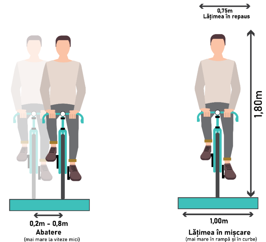
Figură 6-3 - Propunere de dimensionare a infrastructurii de biciclete unidirecționale
