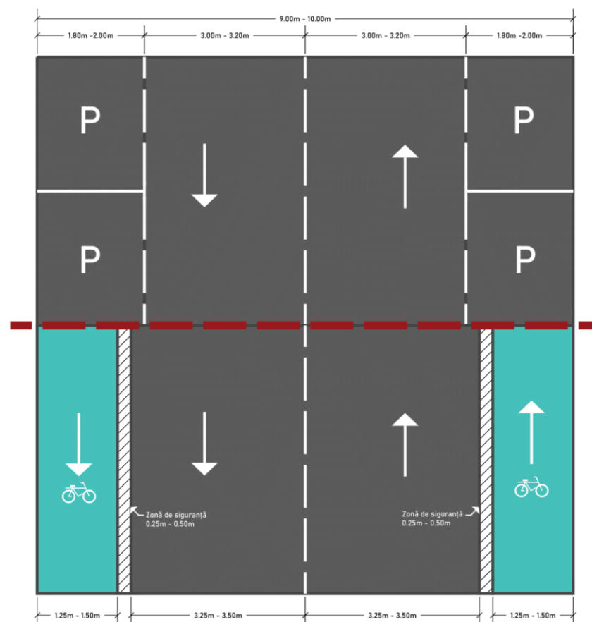
Figură 6-13 - Plan de configurare a unui profil stradal de 9m-10m cu redimensionarea benzilor auto și eliminarea spațiilor destinate parcajului auto și confiugrare de infrastructură velo bidirecțională, respectiv unidirecțională
