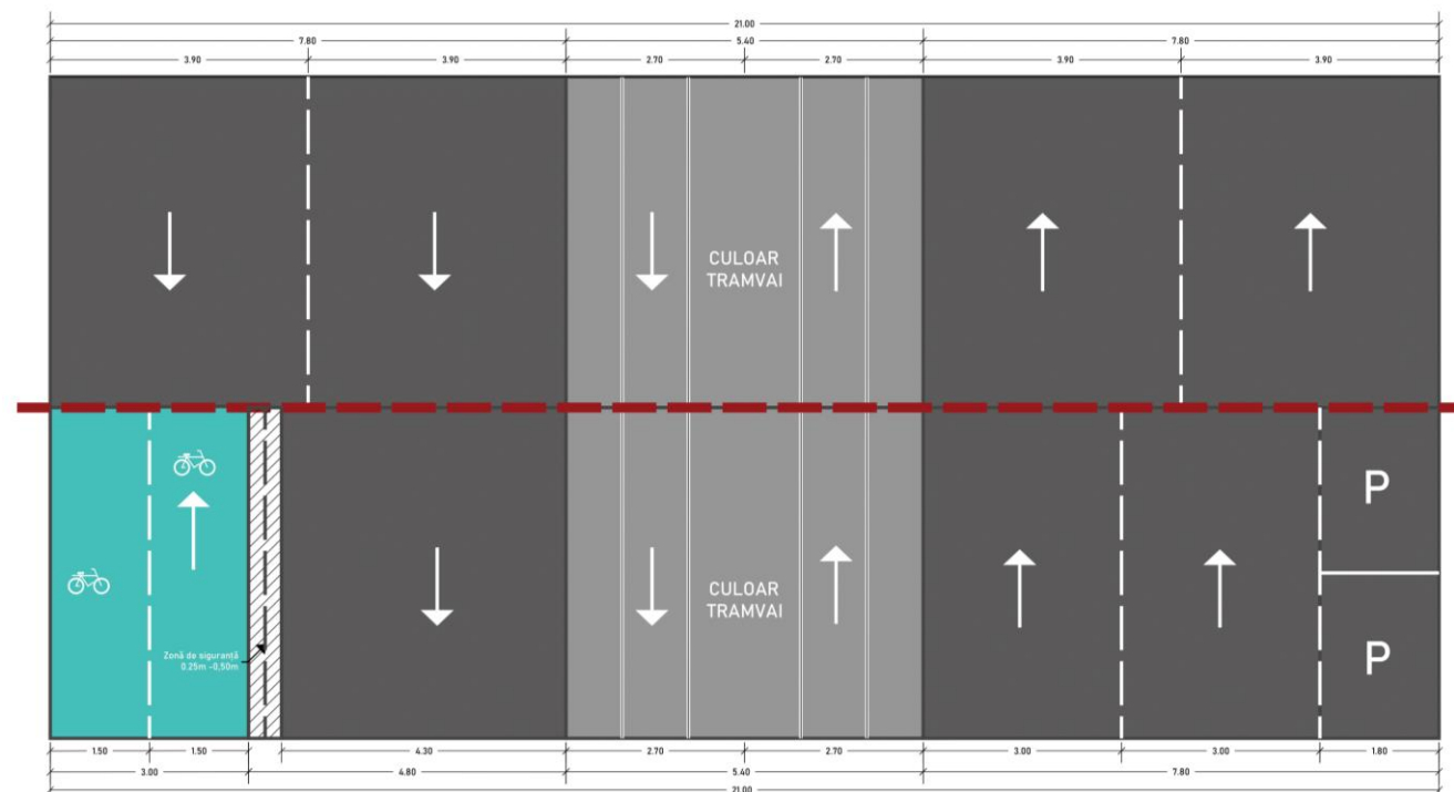
Figură 6-29 - Plan de configurare a unui profil stradal deservit cu culoar de tramvai de 21m cu diminuarea, redimensionarea benzilor auto și configurarea de infrastructură velo bidirecțională din rețeaua principală sau secundară
