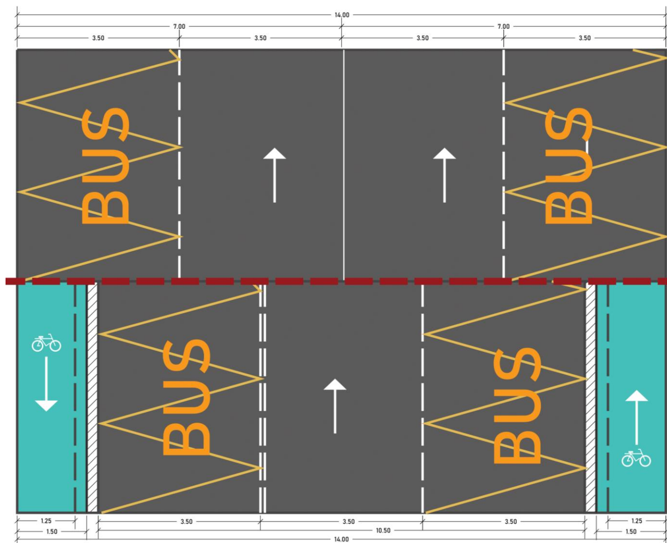
Figură 6-21 - Plan de configurare a unui profil stradal de 14m cu diminuarea și redimensionarea benzilor auto cu pistă unidirecțională pe ambele părți ale spațiului carosabil
