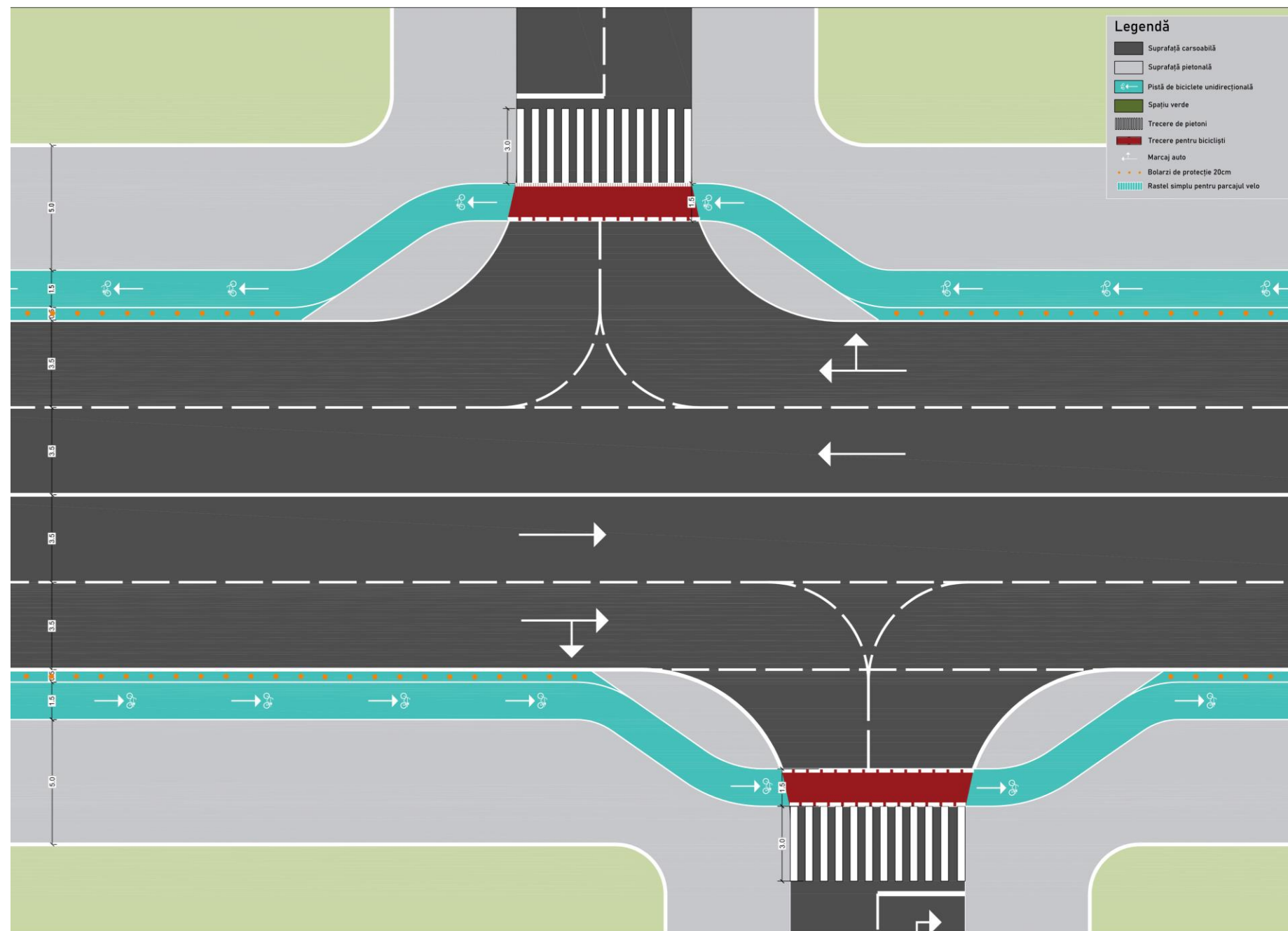
Figură 6-39 - Configurarea unei intersecții rutiere cu traseu de piste de biciclete unidirecționale
