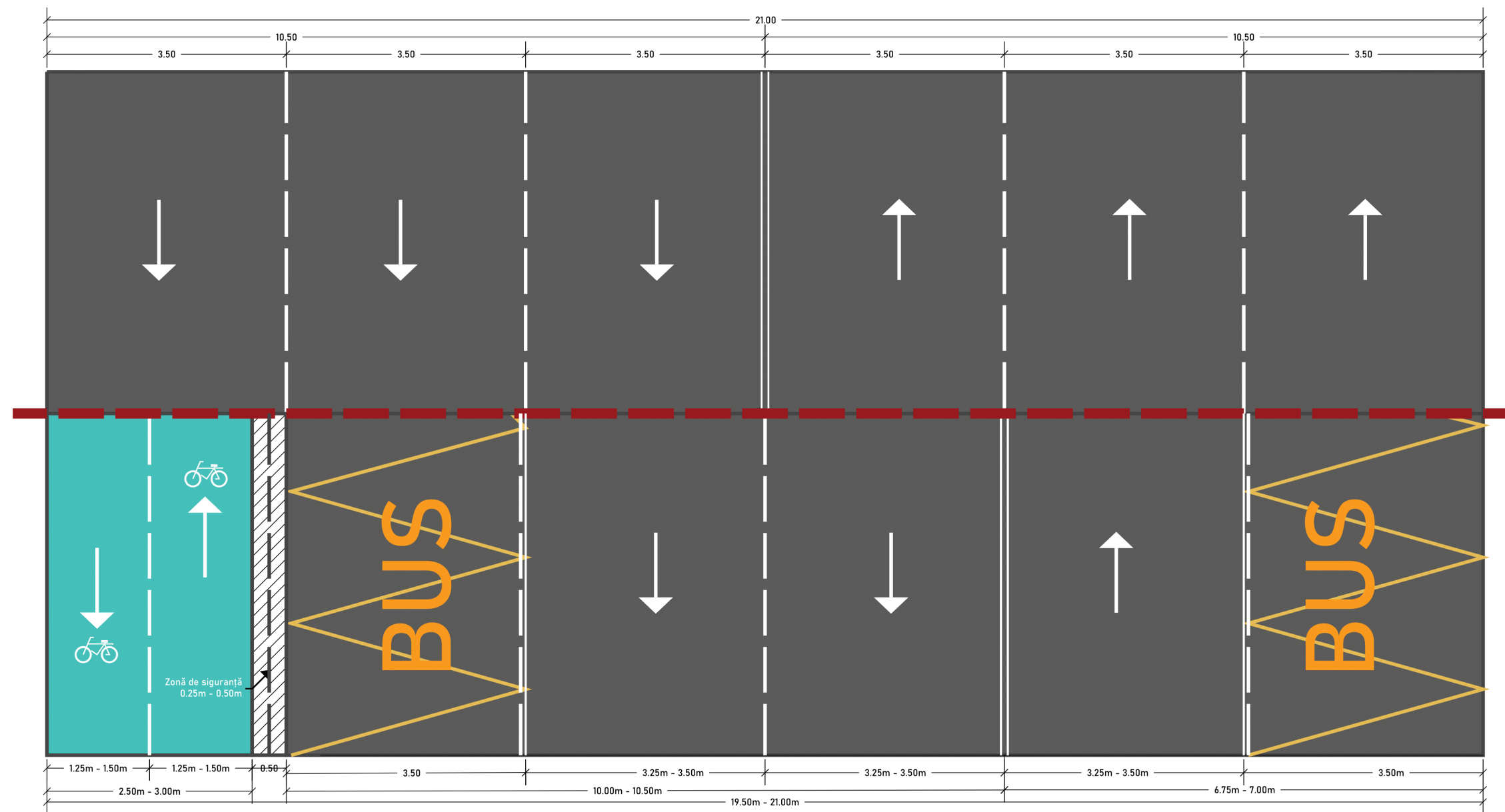
Figură 6-23 - Plan de configurare a unui profil stradal între 21m cu diminuarea, redimensionarea benzilor auto și configurație de infrastructură velo bidirecțională
