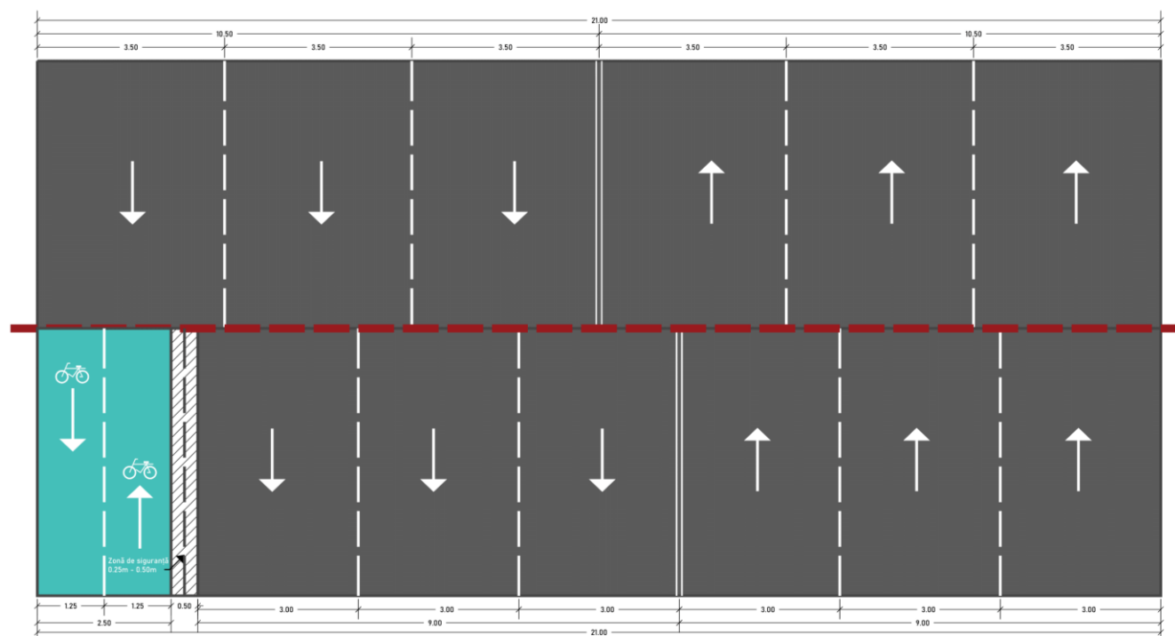
Figură 6-25 - Plan de configurare a unui profil stradal între 21m cu diminuarea benzilor auto și configurarea unei infrastructuri de biciclete bidirecționale
