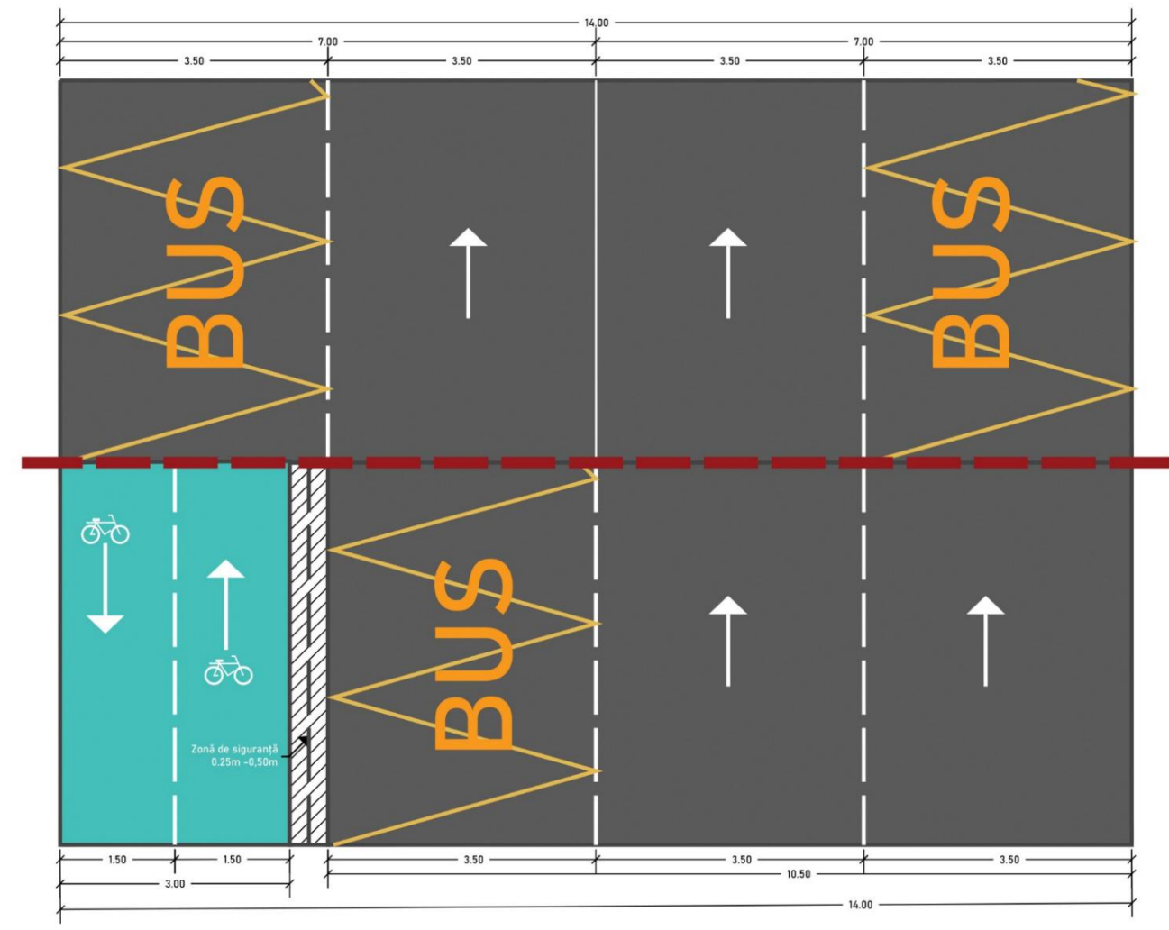
Figură 6-19 - Plan de configurare a unui profil stradal de 14m cu diminuarea respectiv redimensionarea benzilor auto cu pistă bidirecțională pe partea stângă a carosabilului
