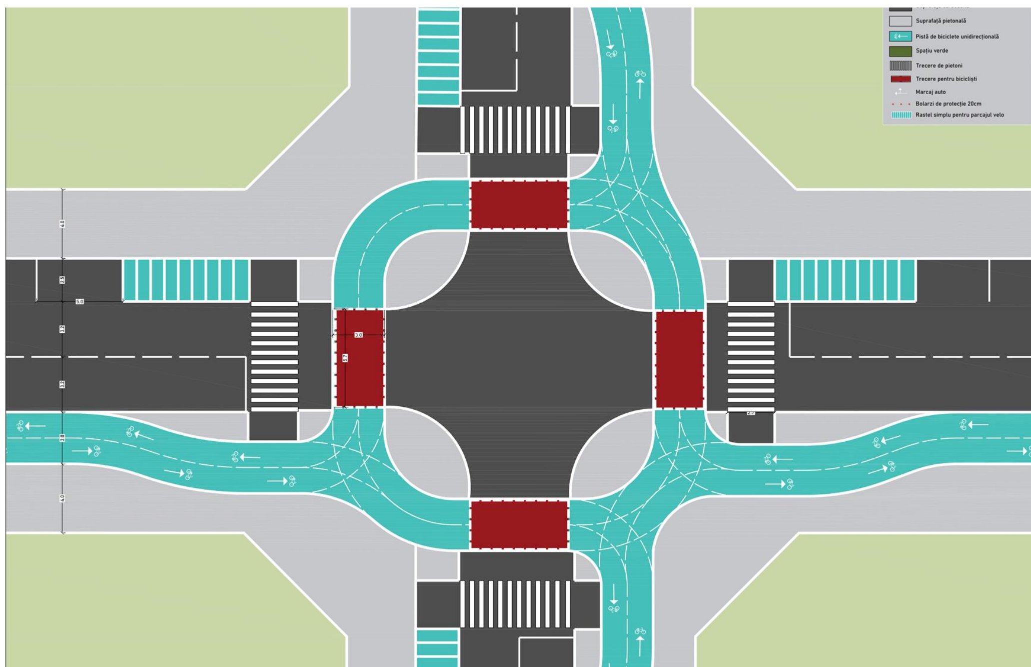
Figură 6-37 - Configurarea unei intersecții rutiere cu traseu de piste de biciclete bidirecționale
