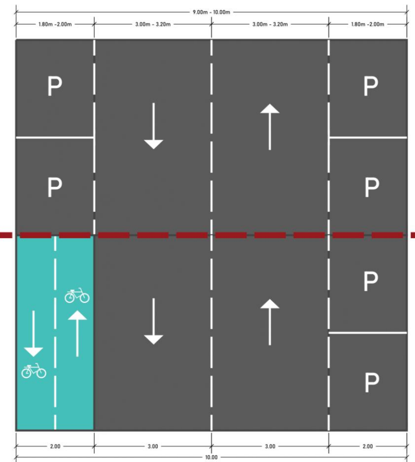
Figură 6-14 - Plan de configurare a unui profil stradal cuprins între 9m și 10m cu restructurarea circulației auto și confiugrare de infrastructură velo bidirecțională respectiv unidirecțională
