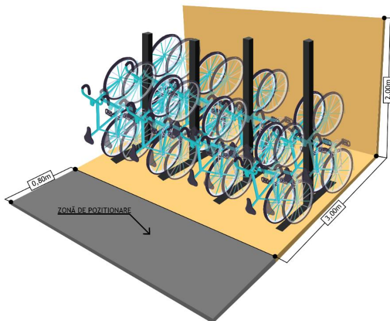
Figură 7-59 - Sistemul de parcare suprapus în cadrul parcajului modular
