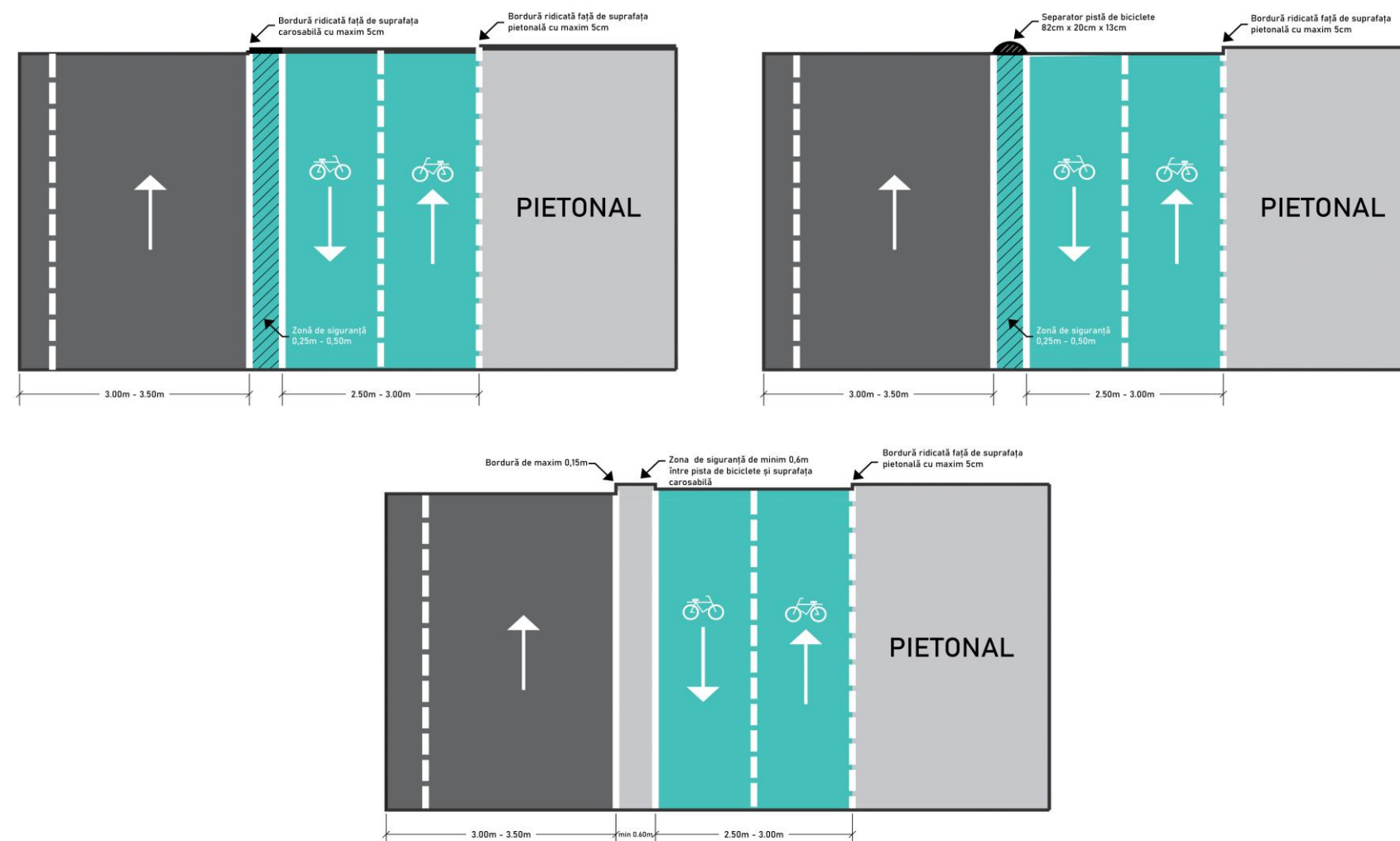
Figură 6-34 - Plan de configurare a zonelor de siguranță aferente pistei de biciclete raportate la suprafața carosabilă respectiv pietonală din imediata proximitate
