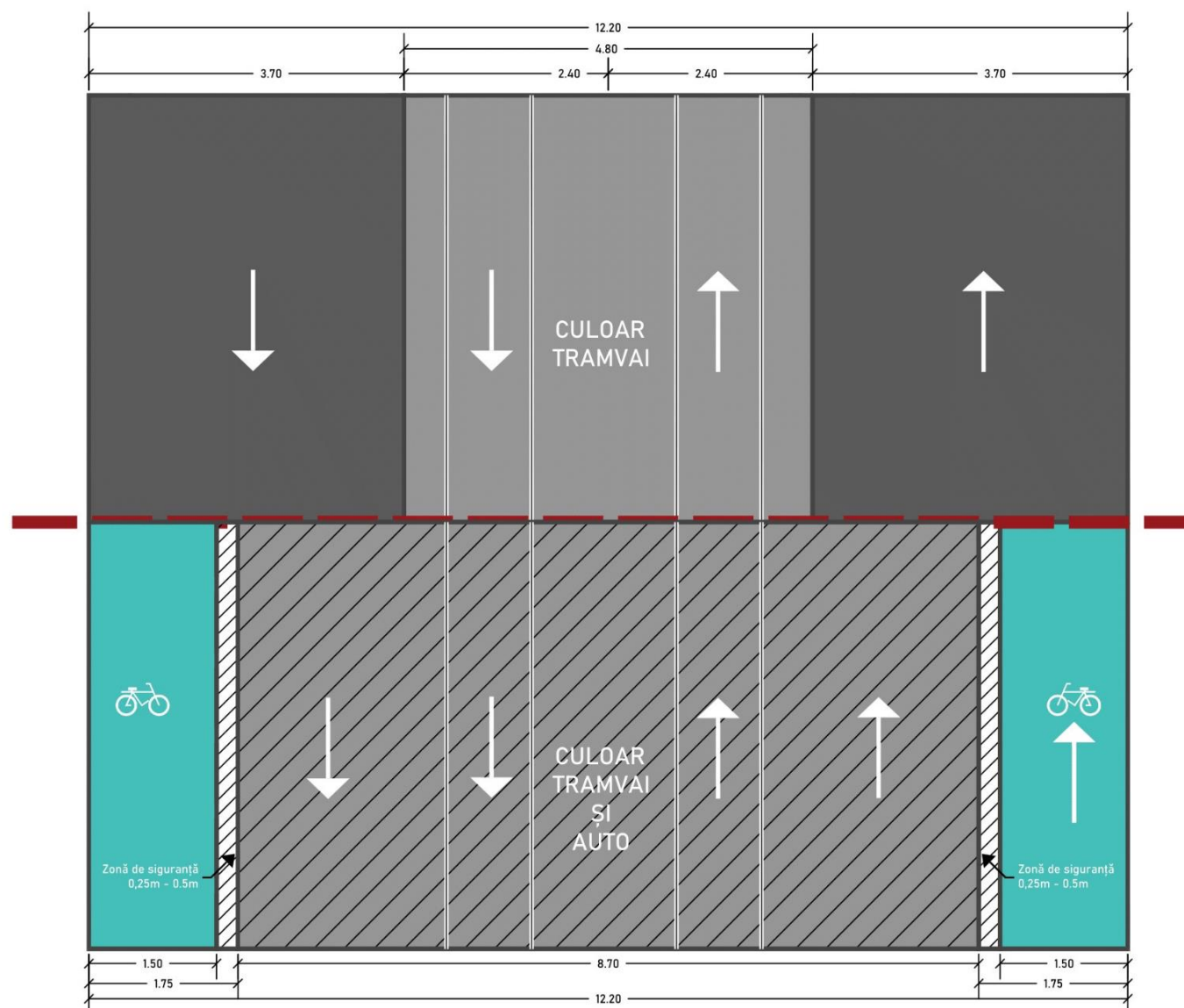
Figură 6-33 - Plan de configurare a unui profil stradal între 12m cu diminuarea respectiv redimensionarea benzilor auto și configurarea unei infrastructuri velo unidirecționale principale
