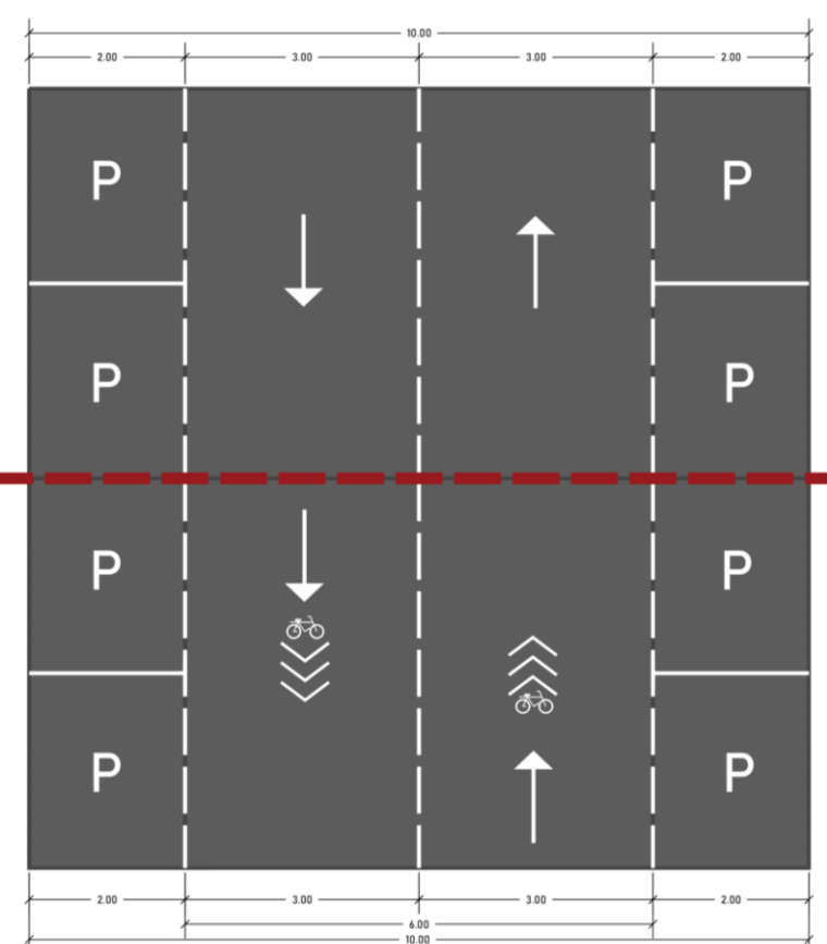
Figură 6-15 - Plan de configurare a unui profil stradal cuprins între 9m și 10m cu restructurarea circulației auto și configuare de infrastructură velo bidirecțională
