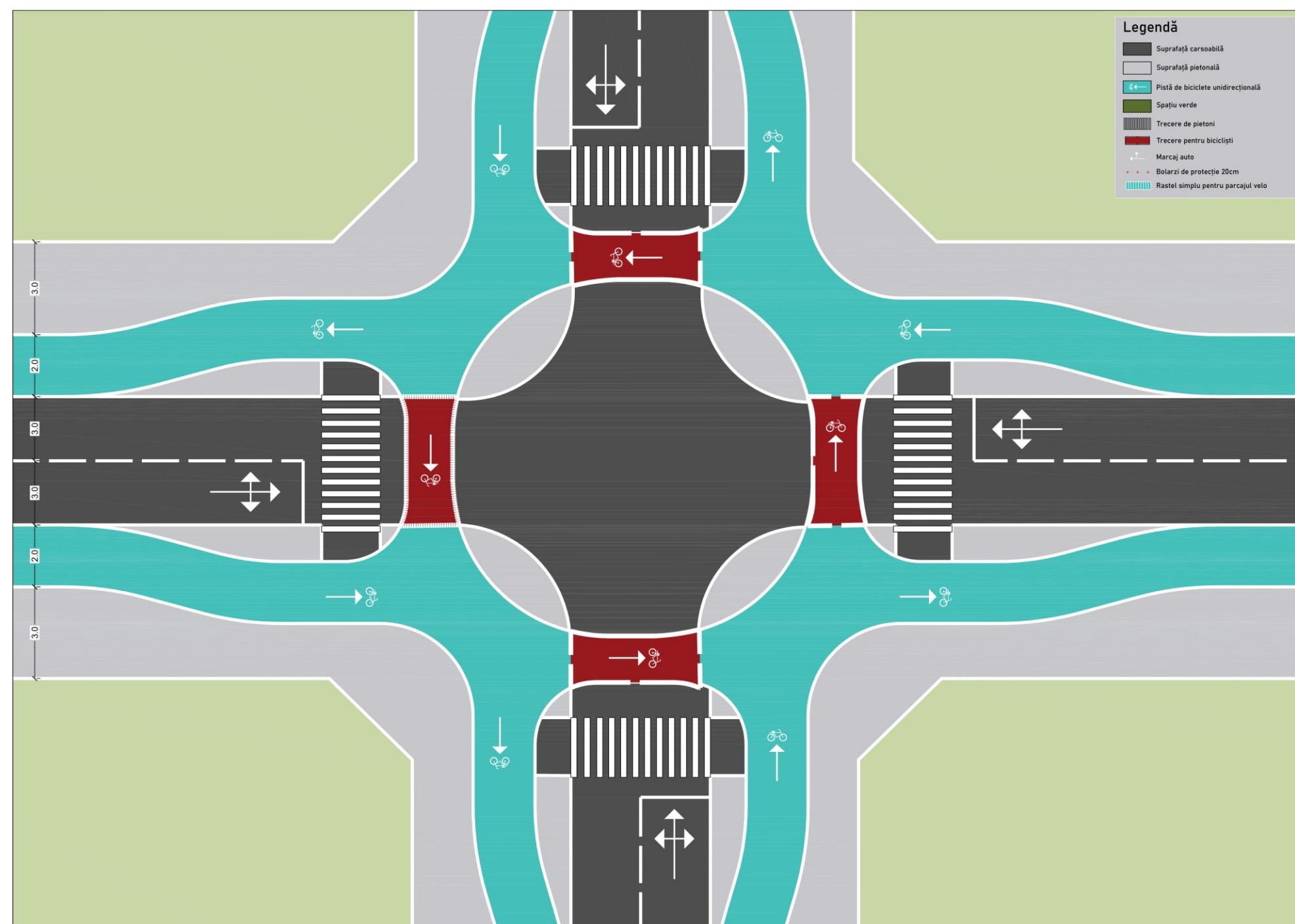
Figură 6-38 - Configurarea unei intersecții rutiere cu traseu de piste de biciclete bidirecționale
