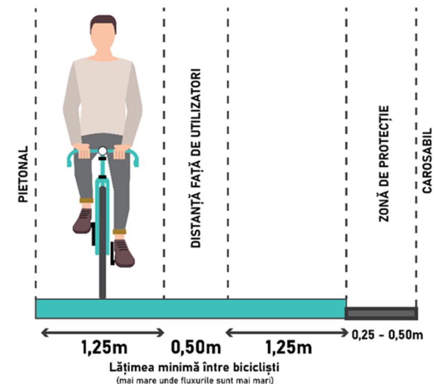
Figură 6-5 - Propunere de dimensionare a infrastructurii de biciclete bidirecționale
