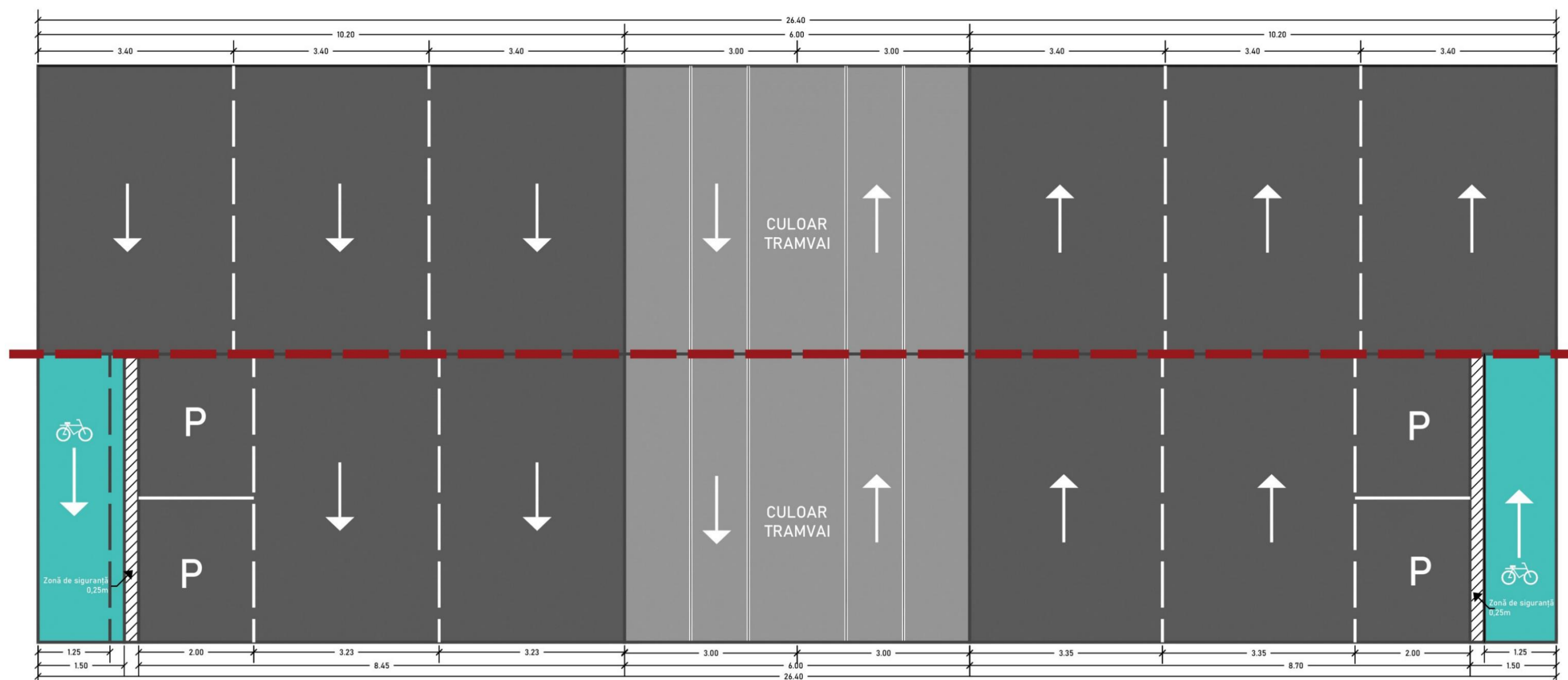
Figură 6-32 - Plan de configurare a unui profil stradal de 26m cu diminuarea și redimensionarea benzilor auto, amenajarea unor spații de parcare a autovehiculelor și configurarea unei infrastructuri velo unidirecționale principale
